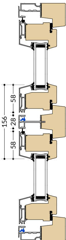
C-C Transom
