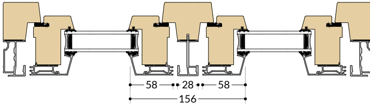
A-A Mullion
